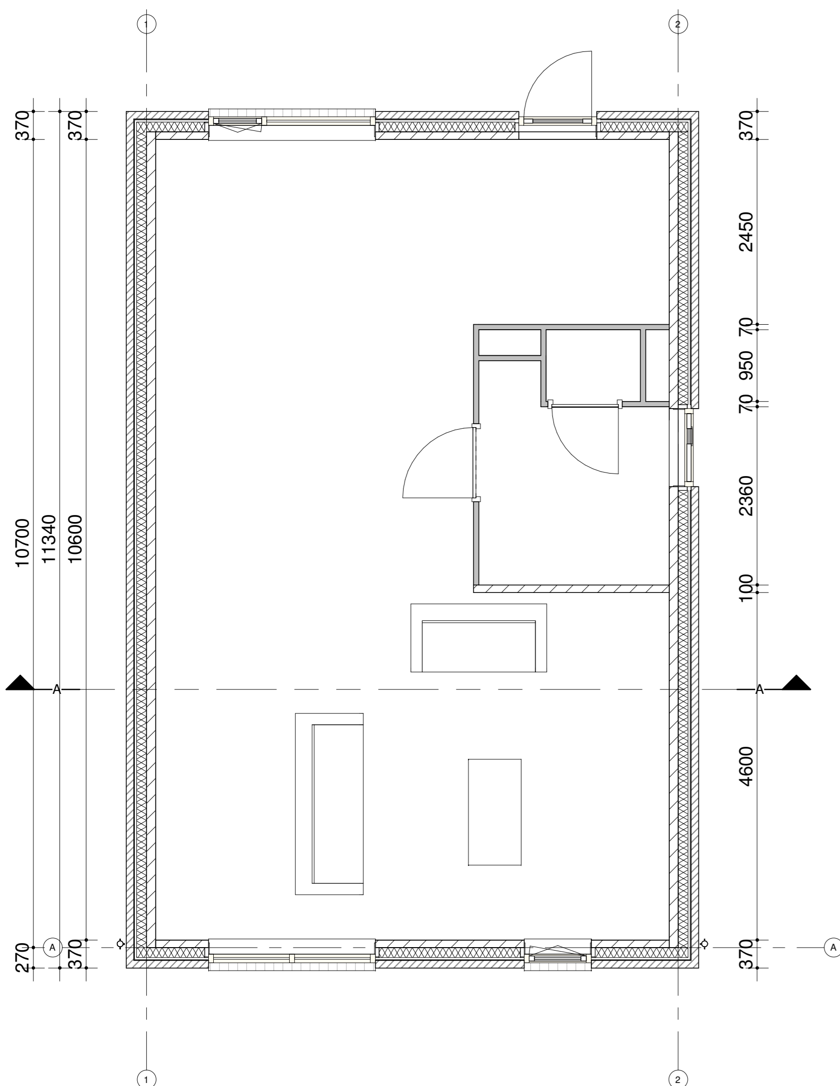
Begane grond
