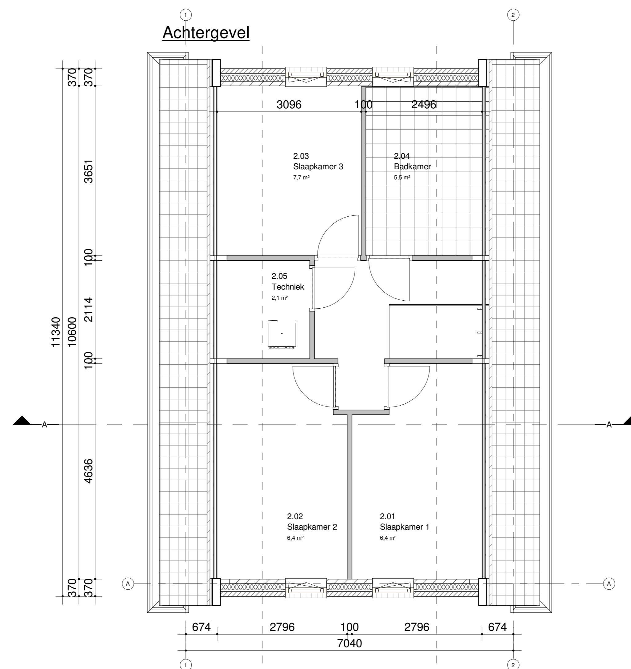
Eerste verdieping
